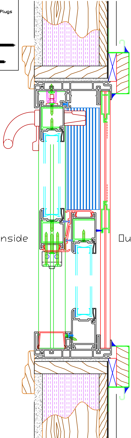
7480 Patio Door Top View
