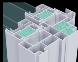
Jamb
